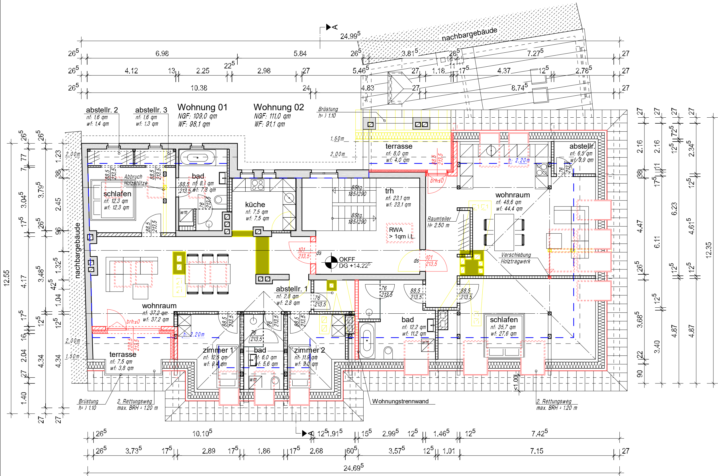
GRUNDRISS 5. obergeschoss
